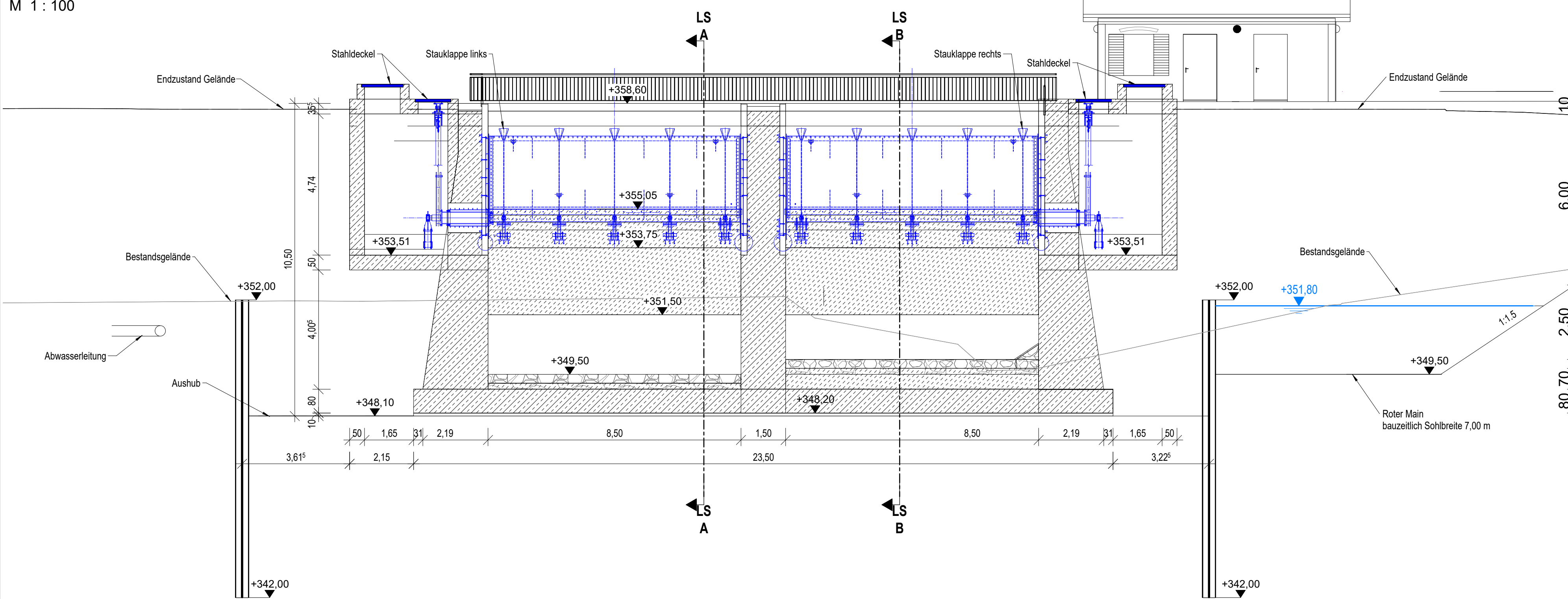
Querschnitt C M 1 : 100
