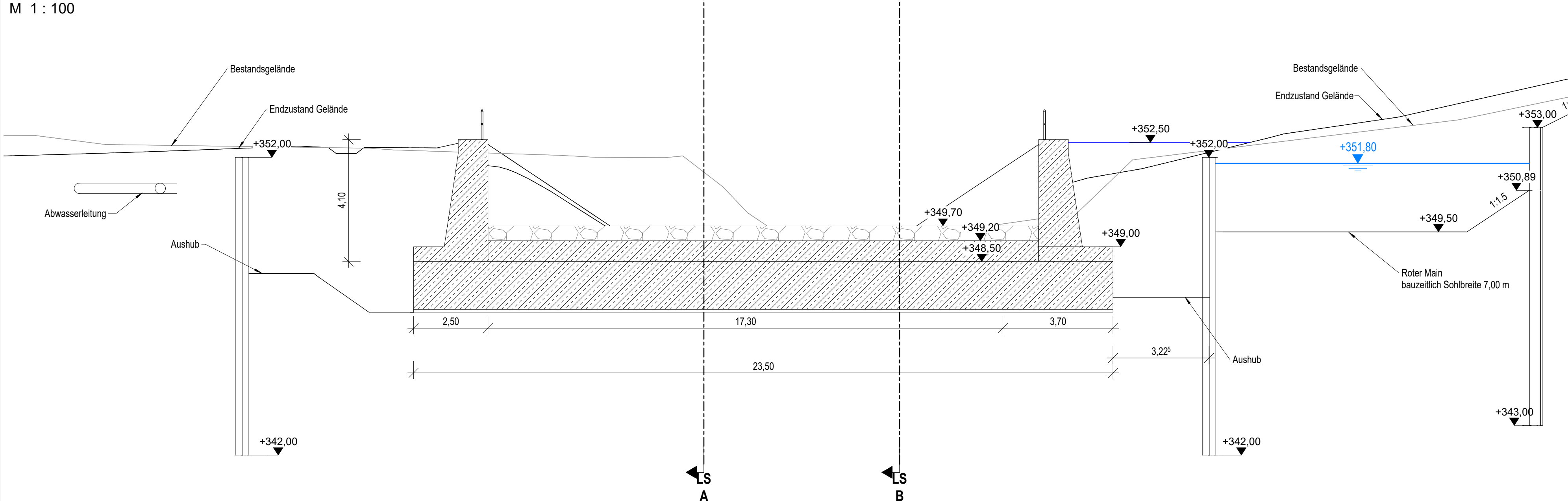
Querschnitt D M 1 : 100
