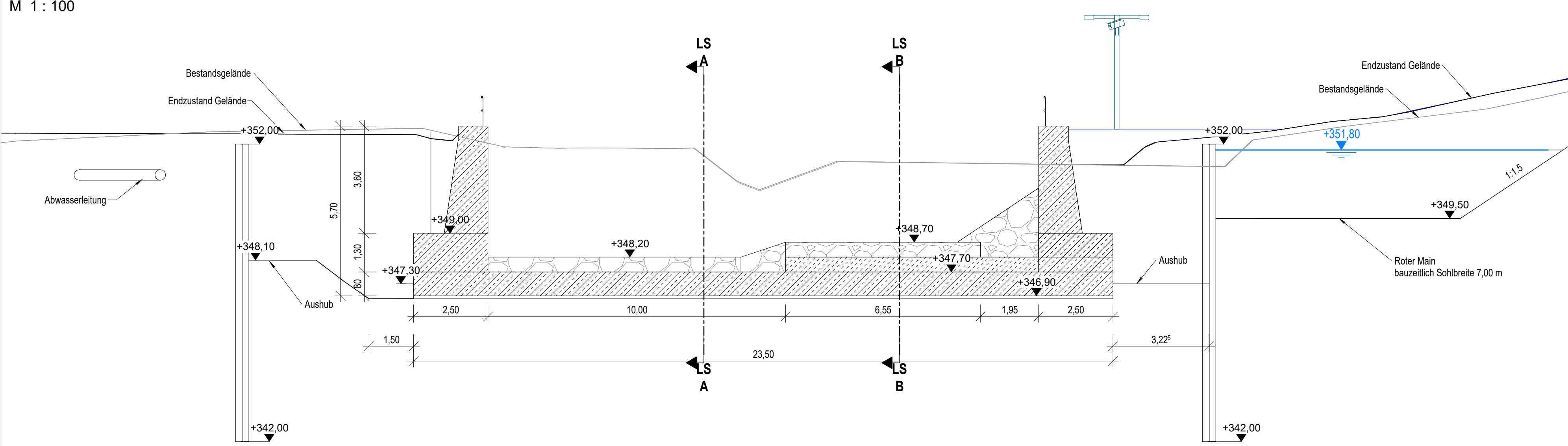
Querschnitt C M 1 : 100
