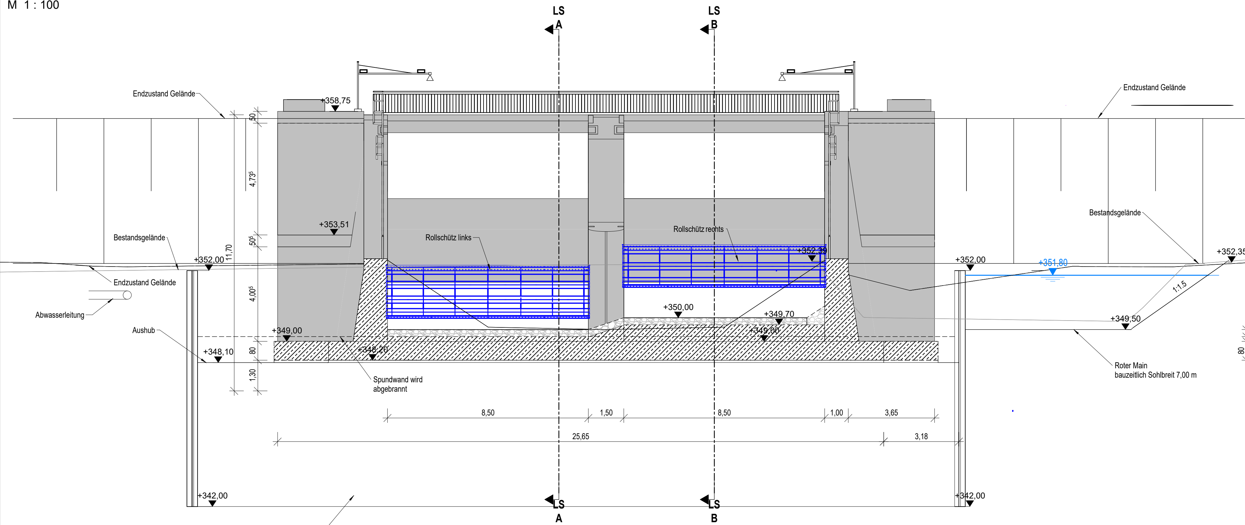
Querschnitt B M 1 : 100
